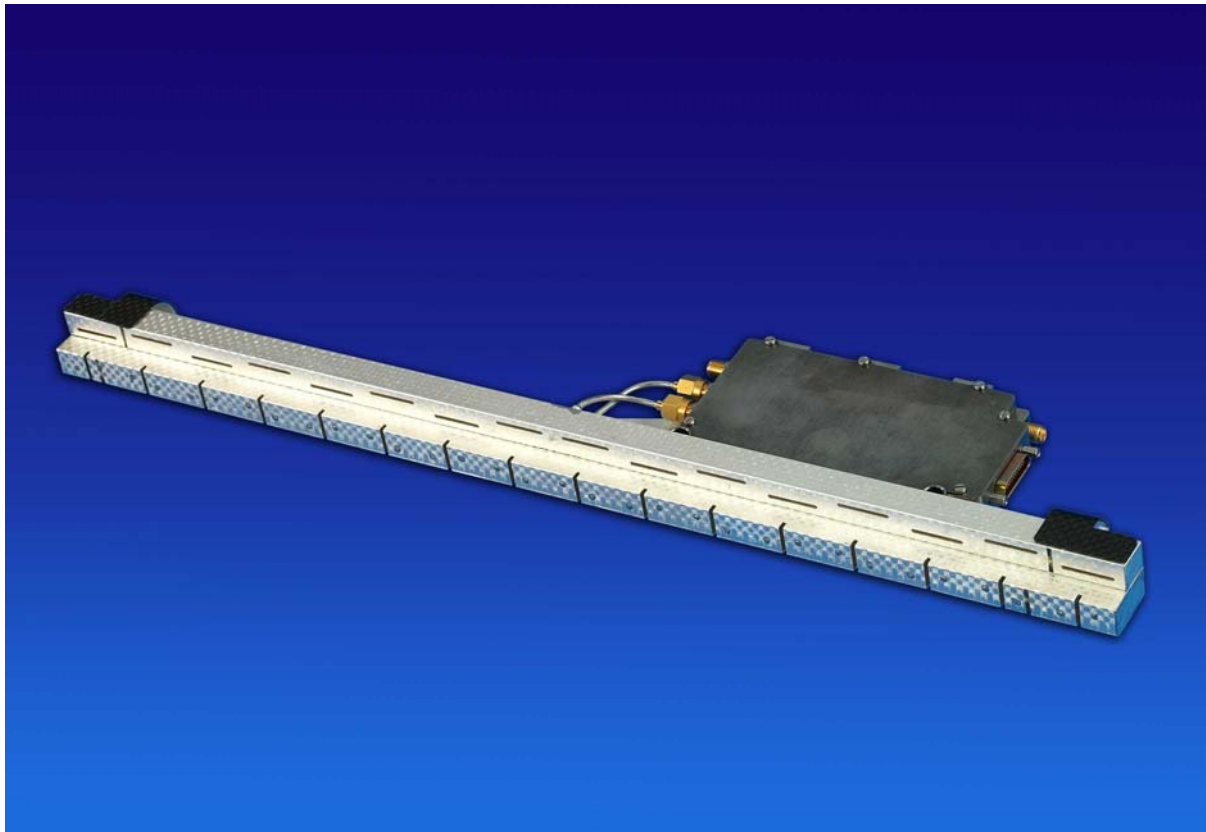
Abb. 14: Subarray mit T/R-Modul, die Querslitze erzeugen die horizontale Polarisierung (HP), die Längsslitze die vertikale Polarisierung (VP)
